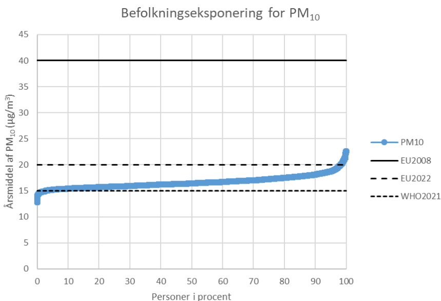
Figur 3.9. Befolkningseksposering for PM 10 i 2019 sammenlignet med grænseværdier og WHO-retningslinjer.
