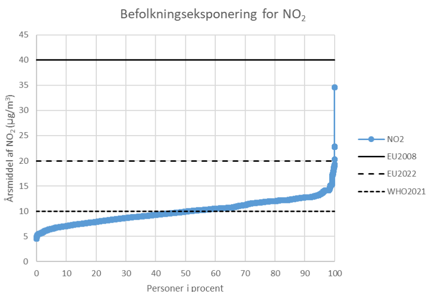
Figur 3.7 Befolkningseksposering for NO 2 i 2019 sammenlignet med grænseværdier og WHO-retningslinjer.
