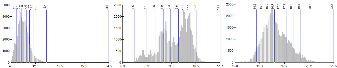
Figur 3.6. Statistisk fordeling af årsmiddelmålinger i 2019 for NO 2 (venstre), PM 2.5 (midte) og PM 10 (højre) langs statsvejnettet. Y-aksen er antallet af observationer og x-aksen er koncentrationsniveauet i µg/m 3 . Blå linjer er baseret på "natural breaks" og svarer til intervalgrænser i figurer, som viser geografiske fordeling.
