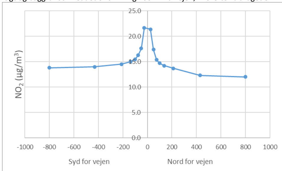
Figur 3.3. Transekt for beregnede årsmiddelværdier af NO 2 i 2019 på strækning på Køge Bugt Motorvejen. Vejens retning er sydvest-nordøst.
