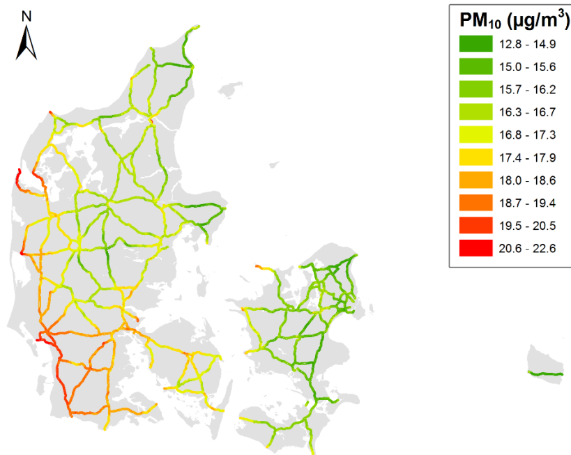
Figur 3.5. Geografisk variation af PM 10 som årsmiddelværdi i 2019 langs statsvejnettet.
