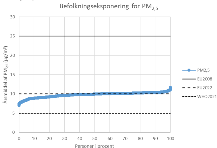
Figur 3.8. Befolkningseksposering for PM 2,5 i 2019 sammenlignet med grænseværdier og WHO-retningslinjer.
