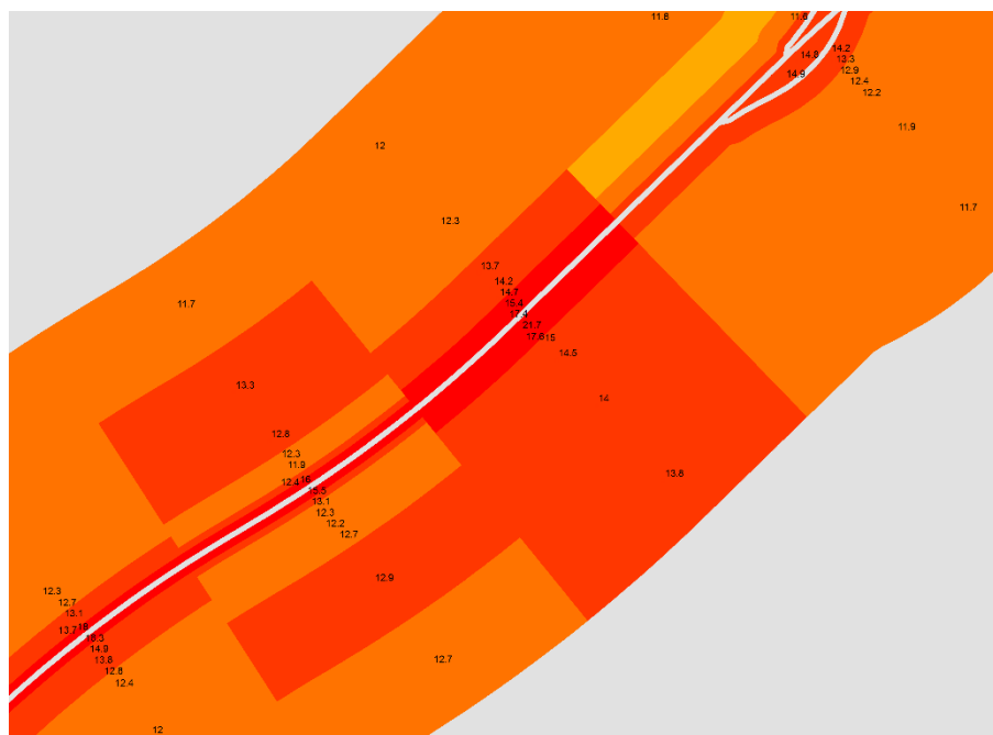
Figur 3.2. Beregnede årsmiddelværdier af NO 2 i 2019 på strækning på Køge Bugt Motorvejen.
