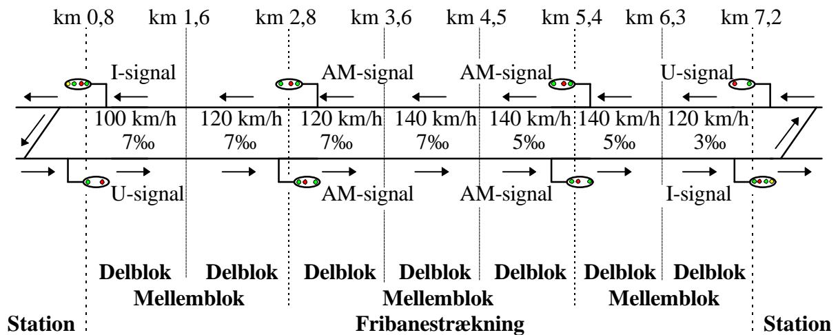
Figur 4 Eksempel på opbygning af en fribanestrækning.
