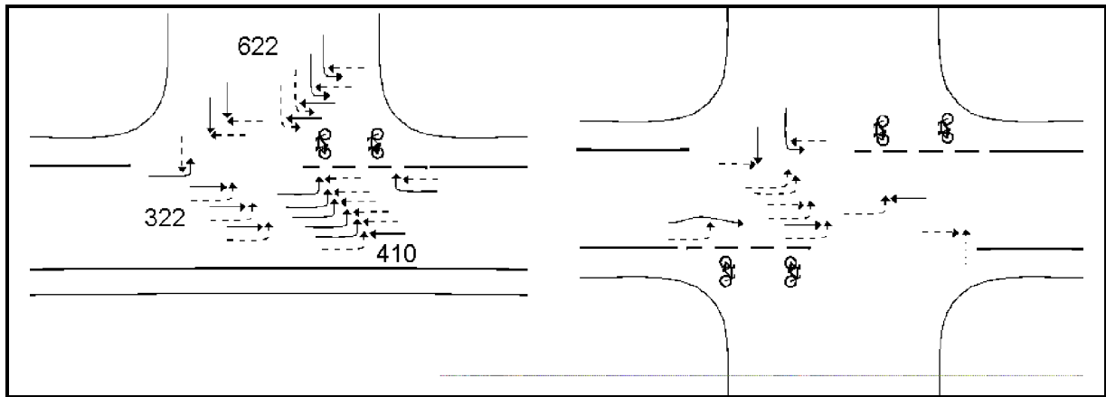
Figur 6 Kollisionsdiagram over uheld med cyklister indblandet i vigepligtsregulerede kryds i efterperioden.
