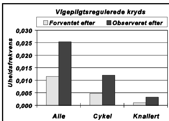
Figur 2 Uheldsfrekvens for uheld i vigepligtsregulerede kryds opdelt på den forventede uheldsfrekvens og den observerede uheldsfrekvens for efterperioden.
