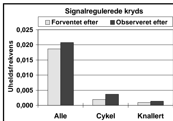
Figur 4 Uheldsfrekvens for uheld i signalregulerede kryds opdelt på den forventede uheldsfrekvens og den observerede uheldsfrekvens for efterperioden.
