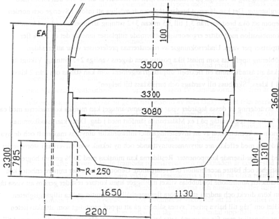
Figur Preliminärt förslag till gemensamt skandinaviskt fordonstvärsnitt för användning i Danmark, Norge och Sverige. Vissa förutsättningar måste gälla;
