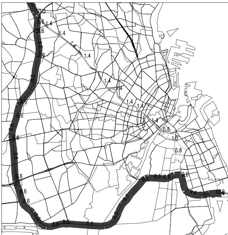
Figur 8. Varebiler i morgenmyldretiden mellem Kbh. Lufthavn og Farum
