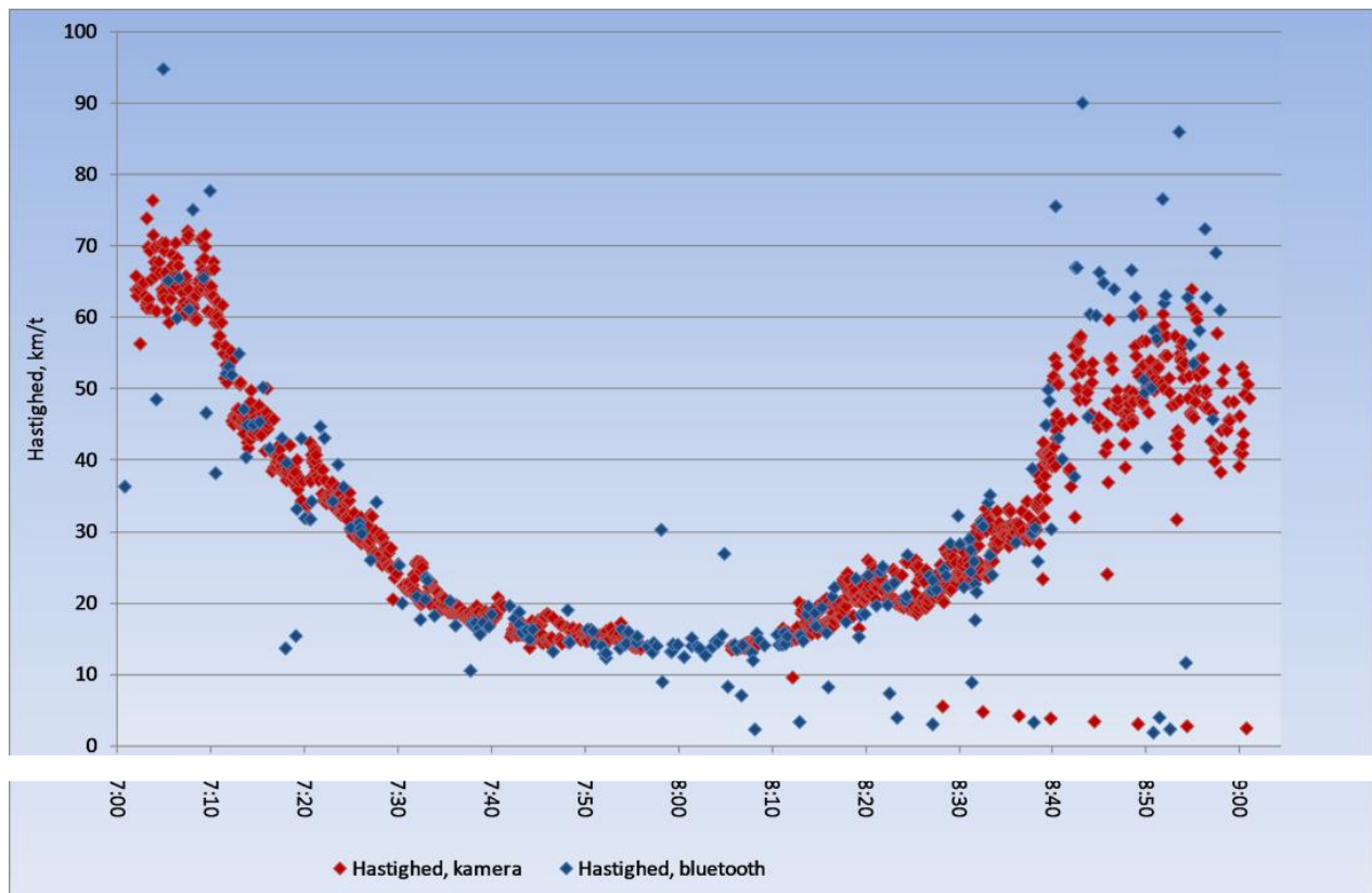
Figur 4: Måling af strækningshastighed med video og Bluetooth
