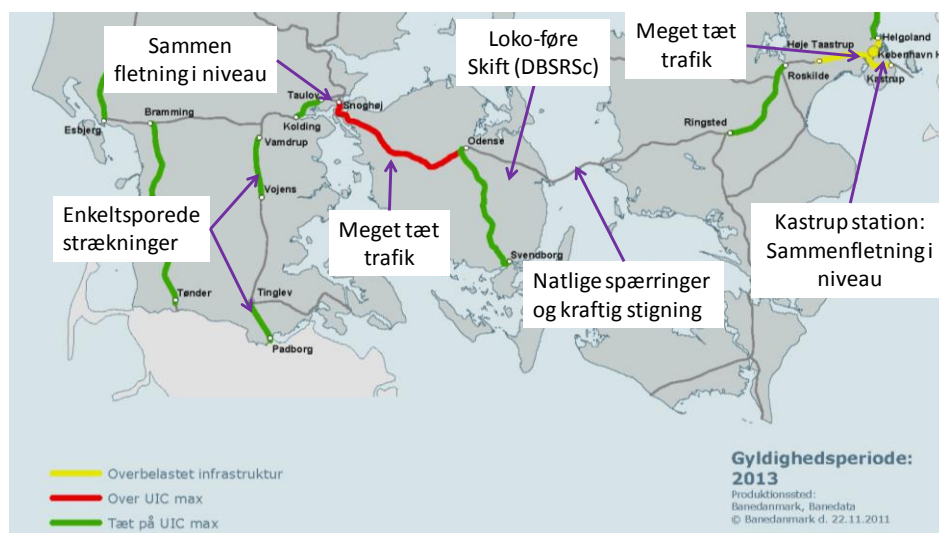
Figur 3: Transitkorridoren Padborg – Peberholm
