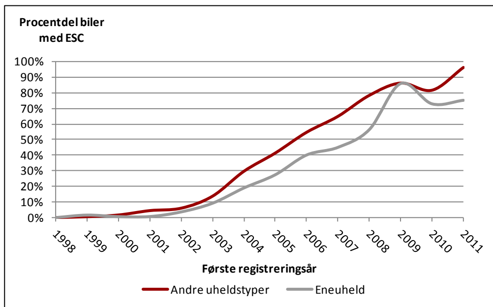
Figur 1. Procentdel af biler i undersøgelsen med ESC installeret i ene- og andre uheld efter første indregistreringsår. N=13.636.
